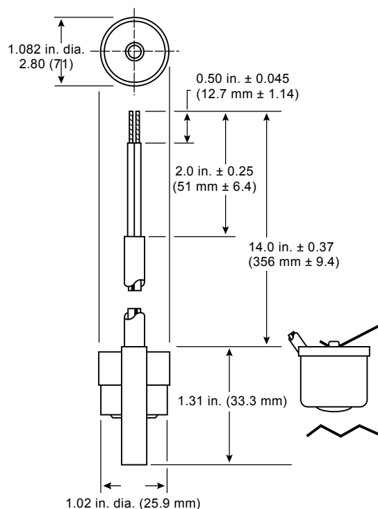
Fig. 14 Aquastat dimensions
